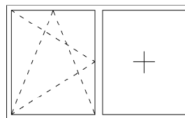
Åpningsvindu med fastfelt
