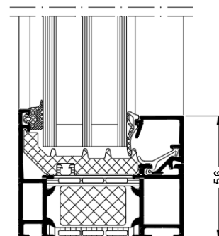
Vertikalsnitt gjennom fastkarm
